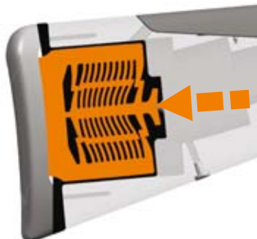
DÉFORMATION AVEC MUNITION MOYENNE Деформация амортизирующих элементов при стрельбе патронами средней мощности
