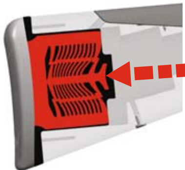
DÉFORMATION AVEC MUNITION LOURDE Деформация амортизирующих элементов при стрельбе мощными патронами
